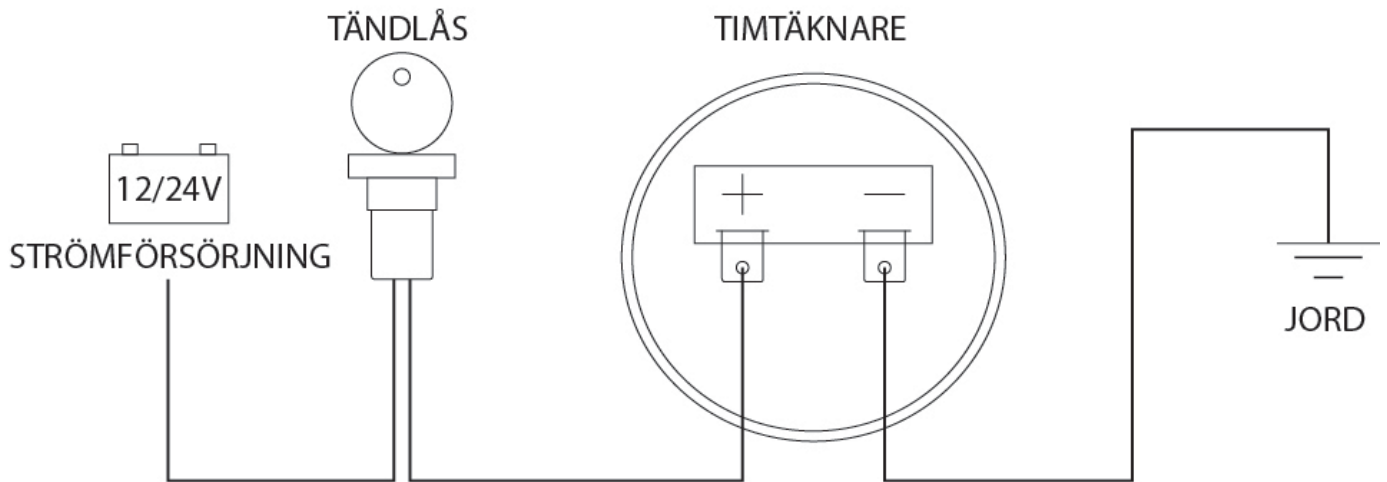
Exempel kopplingsschema
